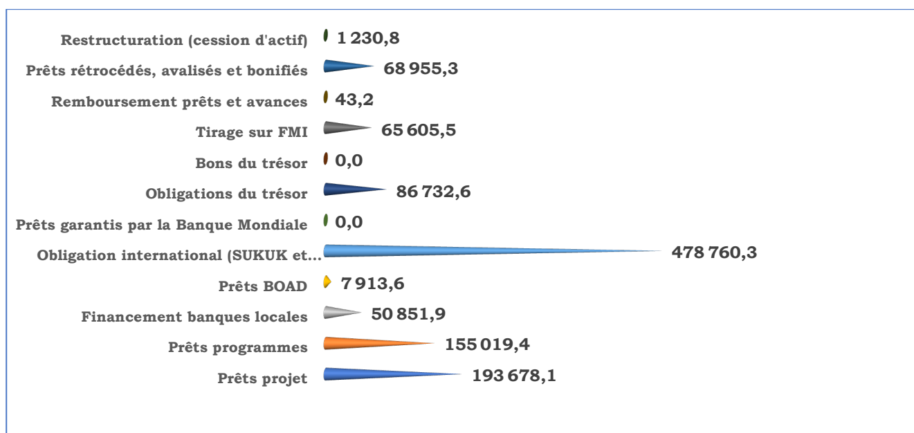
Figure 5 : Niveau d'exécution des nouveaux emprunts au 30 Juin 2026
