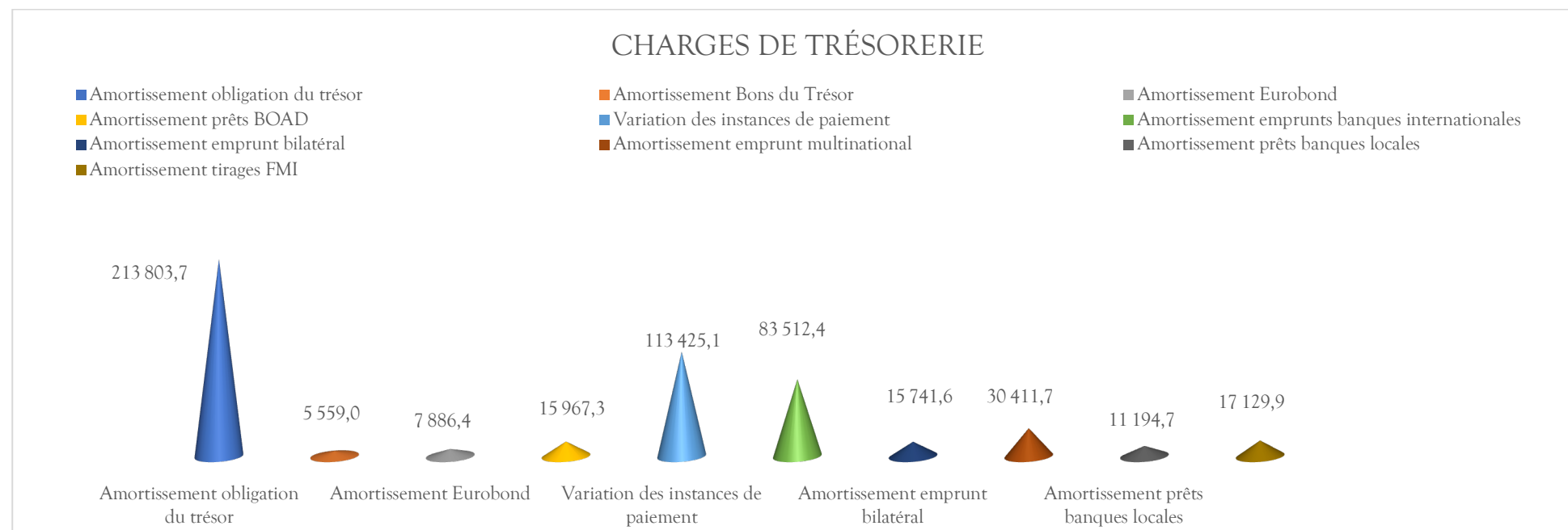
Figure 6 : Niveau de remboursement de la dette passée au 30 Juin 2026
